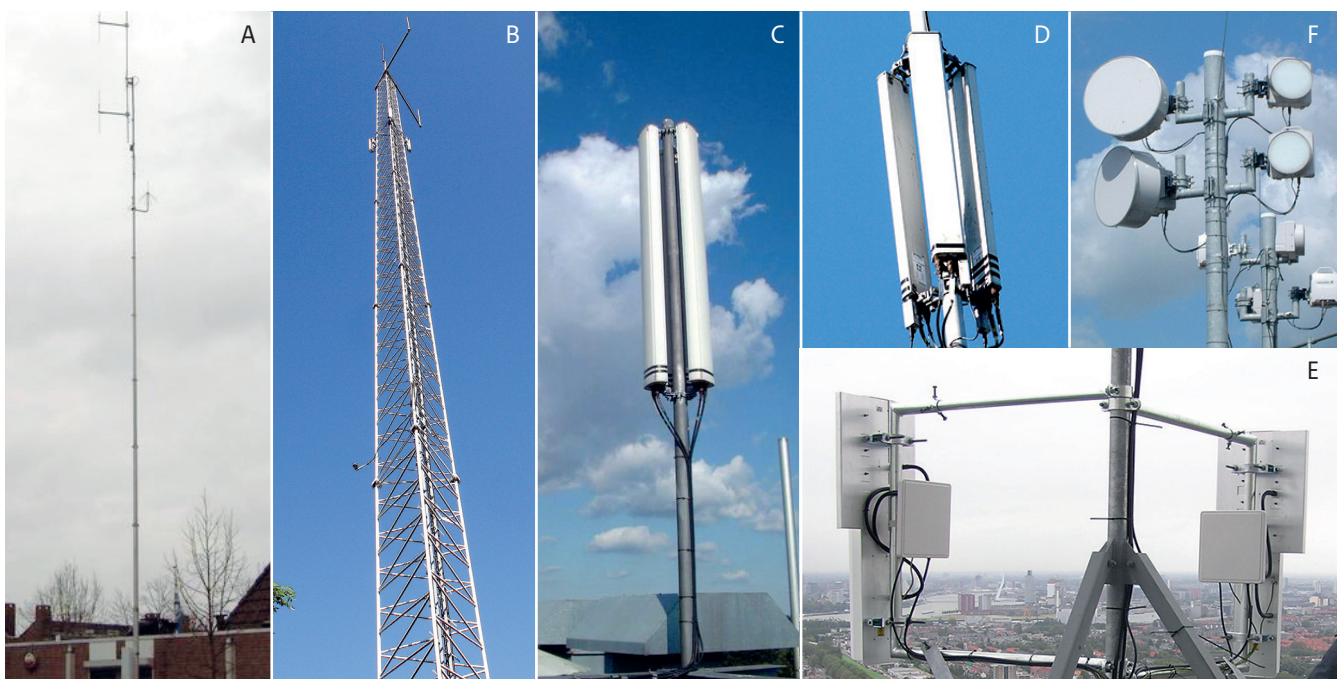
Voorbeelden van veel voorkomende soorten antennes.
